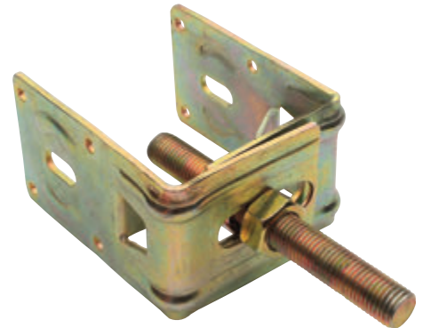
VİDALI PERGÜLE AYAĞI (METAL) SAPLAMA: 14 cm / M16 KOD: 31804
